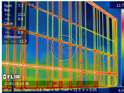
Thermography를 통해 건물 내 개선 부분 해석
